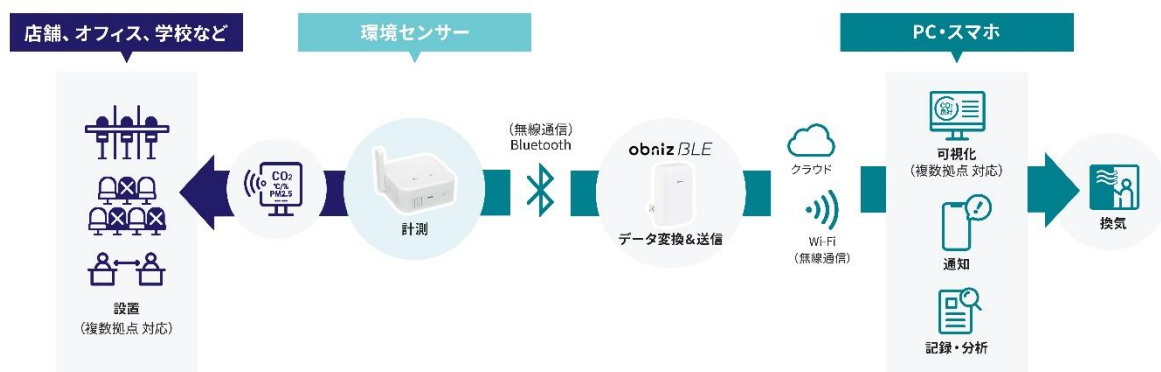
「Sense Connect for 環境監視」計測データの流れ
